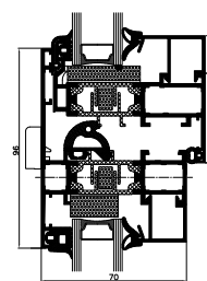
przekrój przez okno otwierane i stałe
