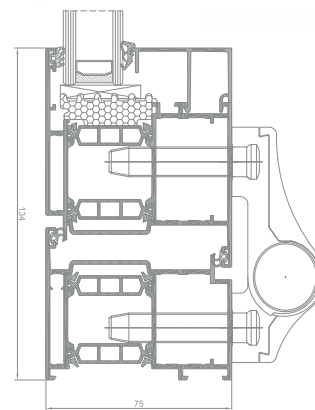
przekrój przez drzwi SP 800 i
