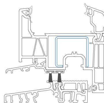
Elegant z ciepłym progiem aluminiowym i zakorągloną listwą - Skala 1:2
